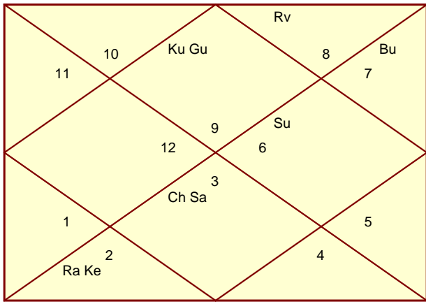
Trimsamsa - Destiny
