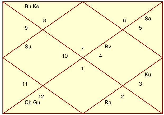
Dasamsa - Profession
