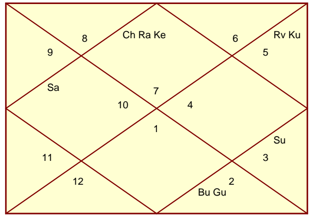
Khavedamsa - Auspicious
